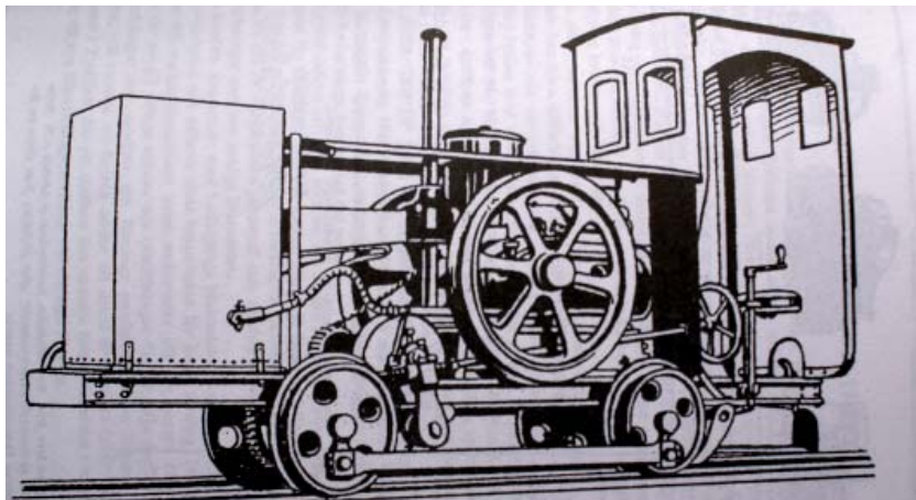
Lok 2. Motorlokomotivet Warant. Det största lokomotivet hade en motor på 16 hästkrafter och vägde 3 400 kilo. Priset var enligt en priskurant 6.500 kronor.
